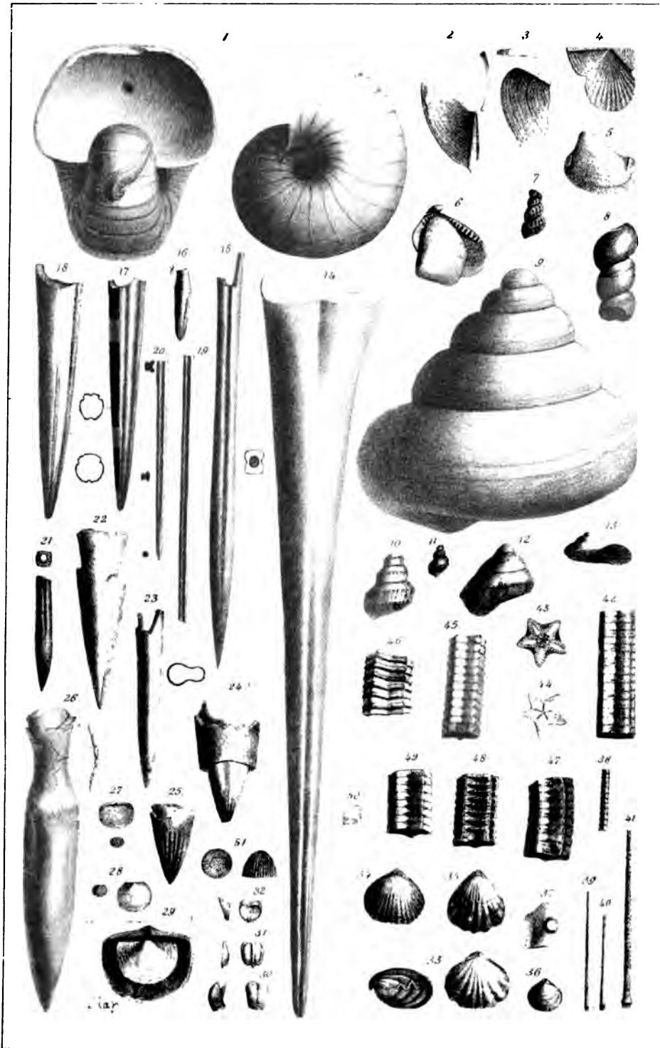
Ammonit. Lib.
